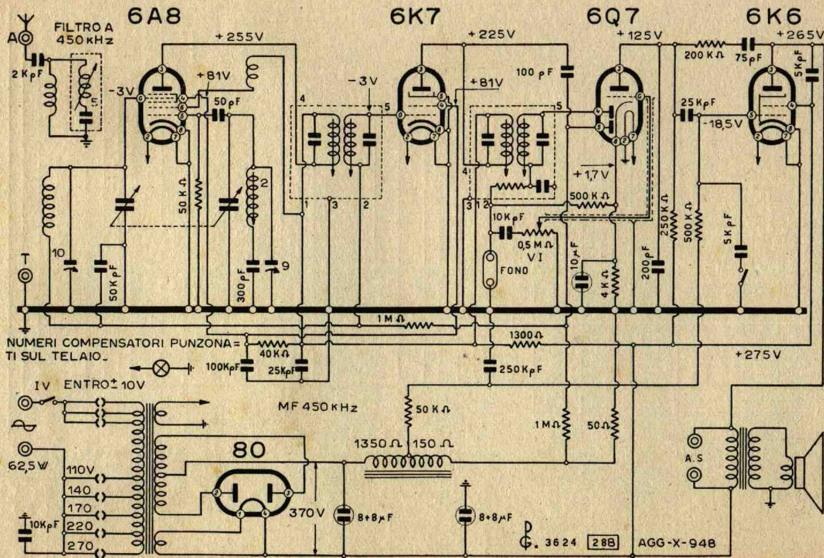
Lo schema elettrico del Mono-Unda 511.
